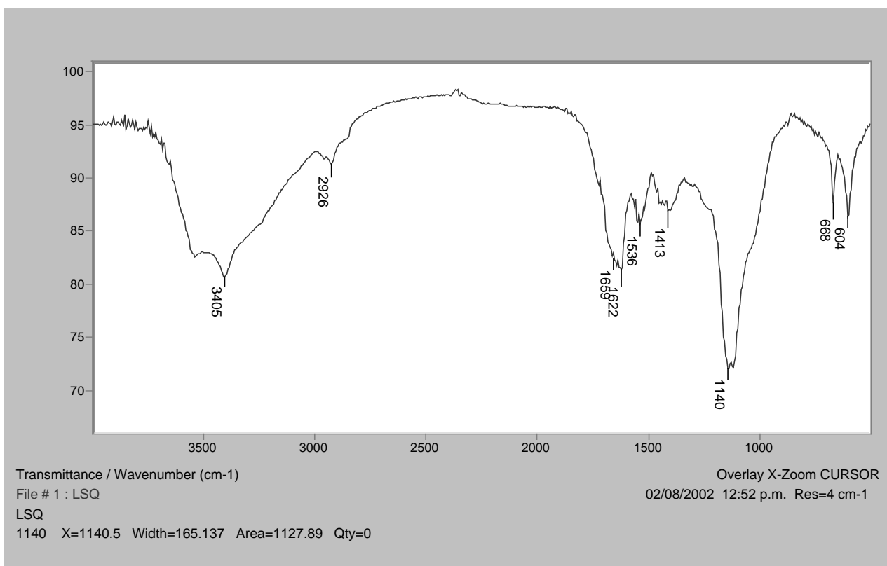
Fig.5. Espectro infrarrojo de la muestra sin azufre.
