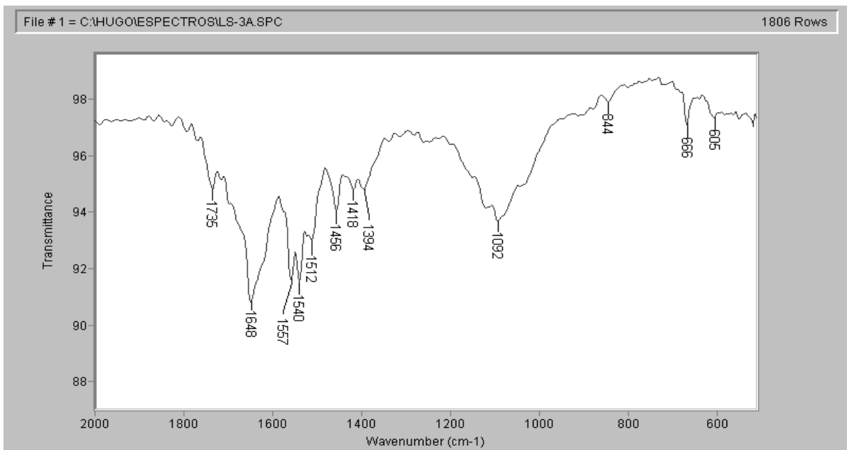
Fig.4. Espectro Infrarrojo de la muestra en polvo.
