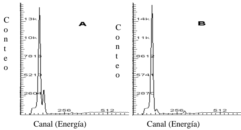
Fig. 3. Espectro fotoelectrónico de rayos x. A patrón de azufre y B muestra.
